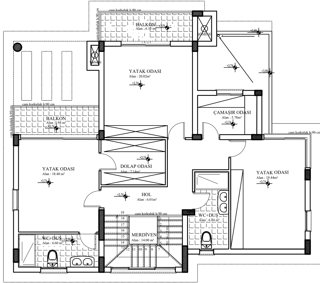
E BLOK BİRİNCİ KAT PLANI ÖLÇEK:1/50
